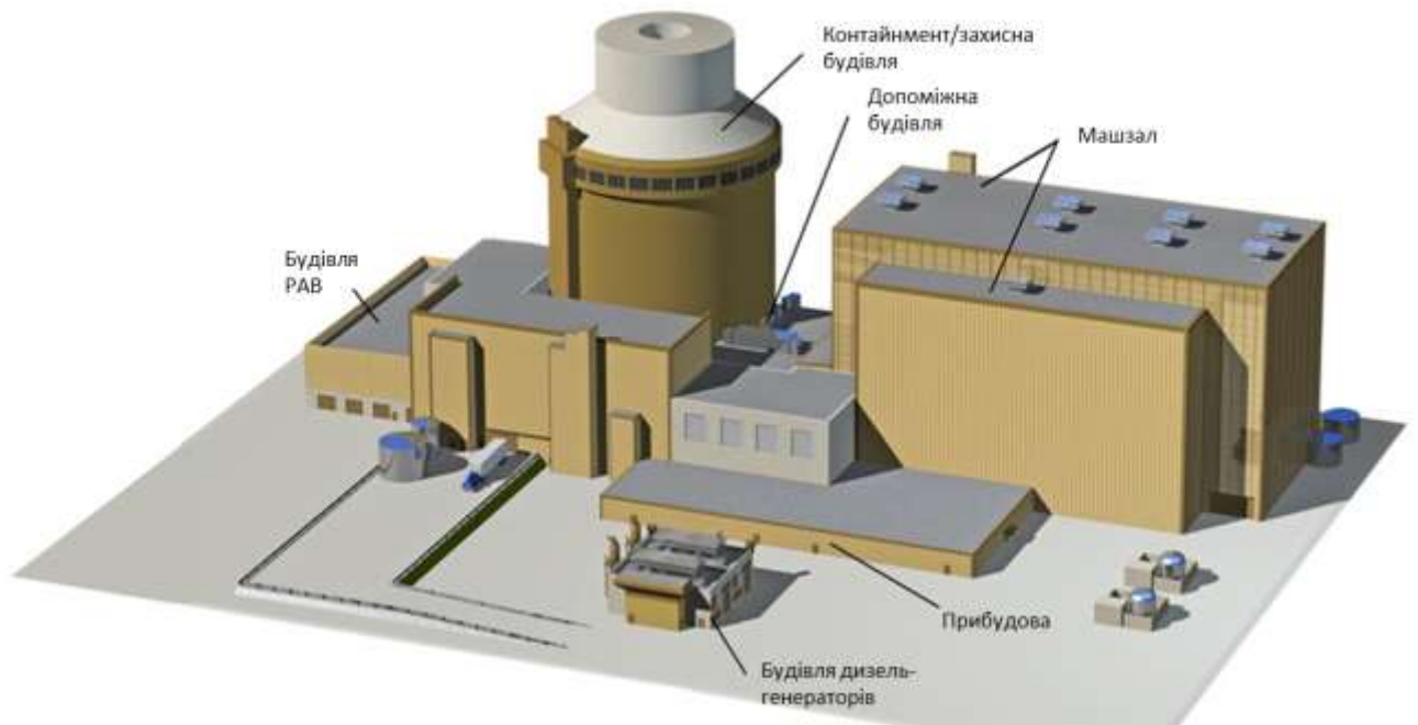
Рисунок 1.2 – Енергоблок AP1000
