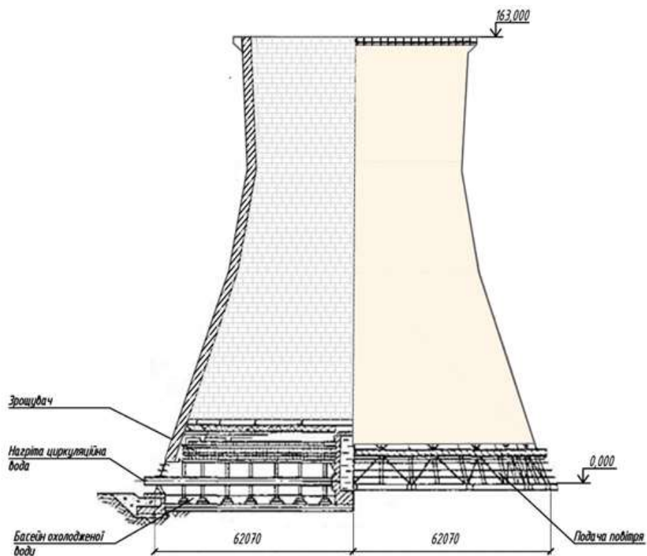
Рисунок 5.1 – Баштова градирня
